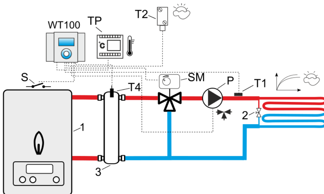
Hydraulické schéma s třícestným ventilem regulujícím okruh podlahového vytápění (s hydraulickou spojkou) 3
