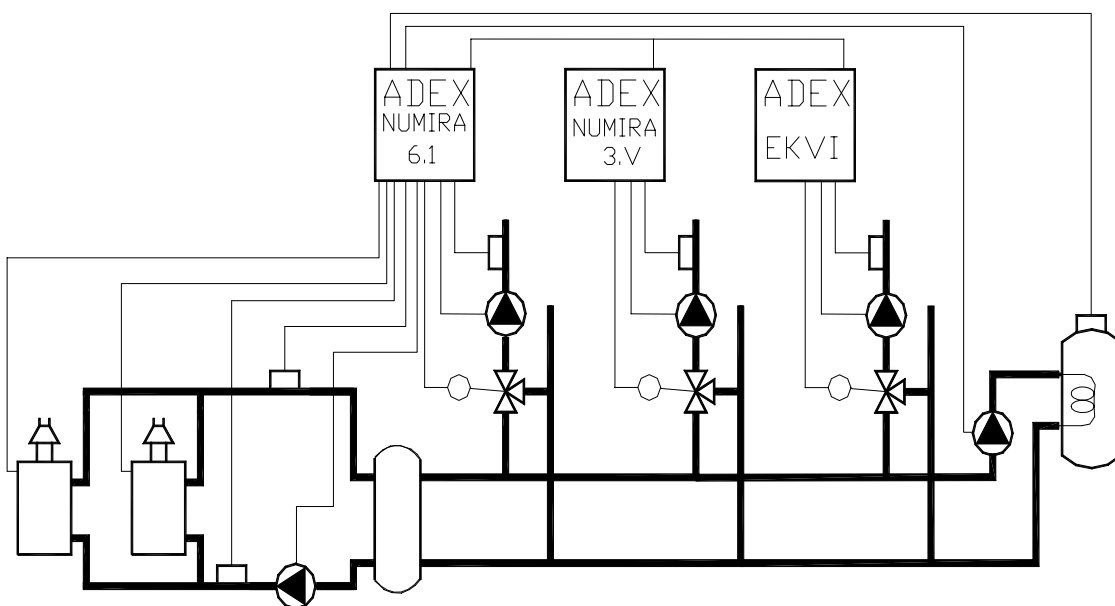
Příklad řešení kotelny s anuloidem a rozvětveným systémem
