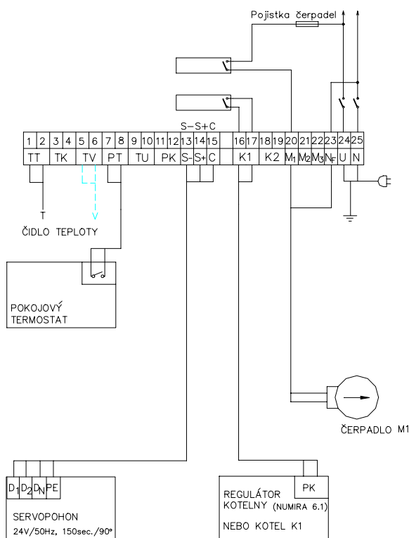
Příklad řešení kotelny s anuloidem a rozvětveným systémem
